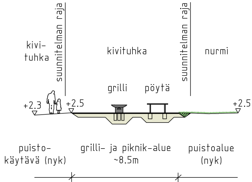
LEIKKAUS A-A, 1:200
